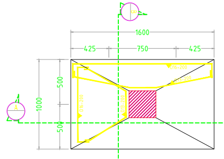
DENAH PONDASI P2 SKALA 1 : 25
