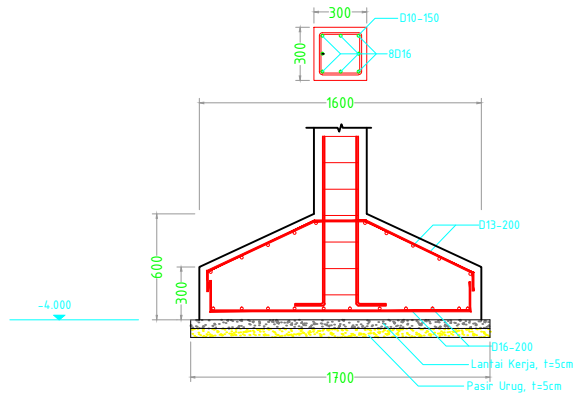
POTONGAN A SKALA 1 : 25
