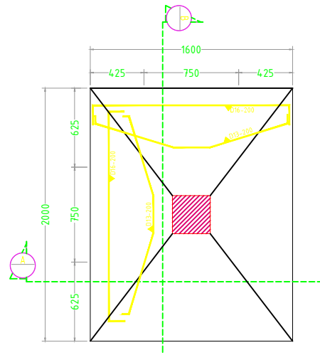
DENAH PONDASI P1A SKALA 1 : 25
