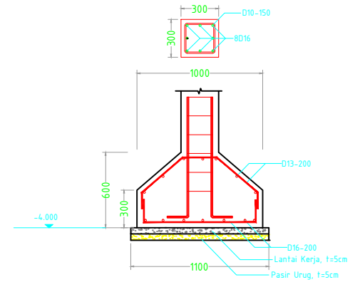
POTONGAN B SKALA 1 : 25
