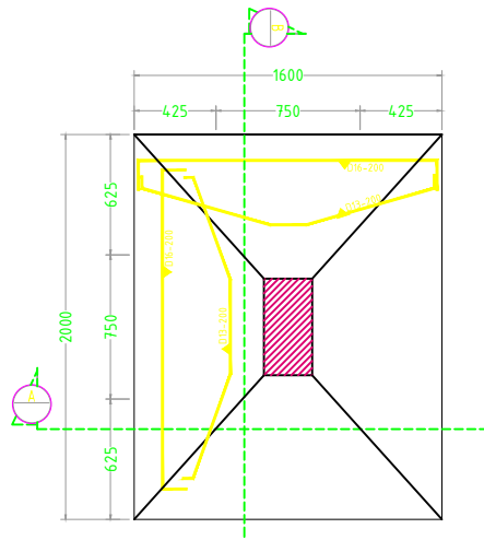
DENAH PONDASI P1B SKALA 1 : 25
