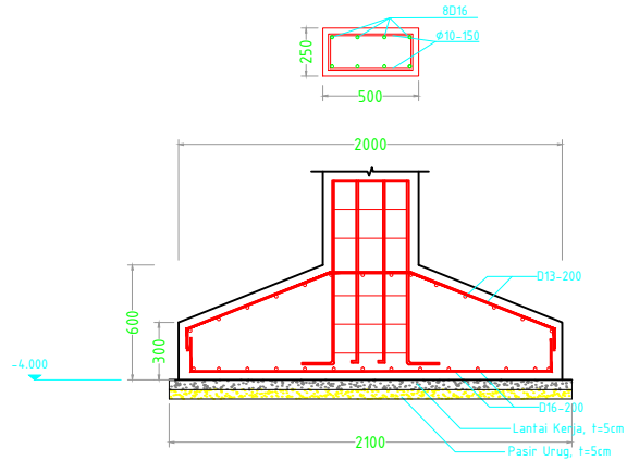
POTONGAN B SKALA 1 : 25
