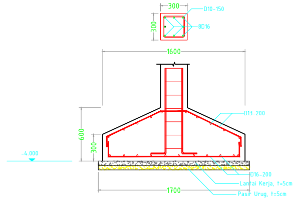
POTONGAN B SKALA 1 : 25
