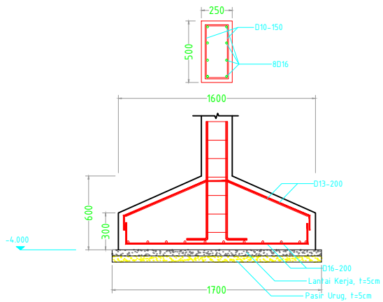
POTONGAN A SKALA 1 : 25
