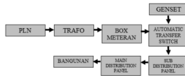
Gambar 14. Arus Listrik
