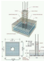
Gambar 19. Pondasi
