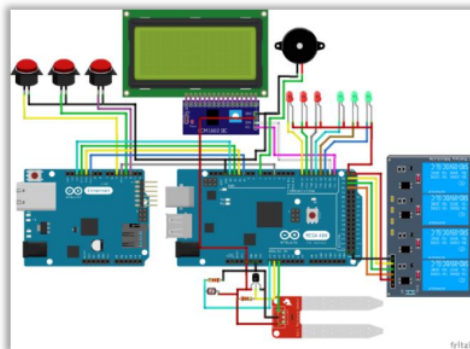
Gambar 8. Rangkaian keseluruhan sistem
