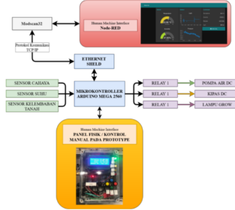
Gambar 7. Diagram blok sistem
