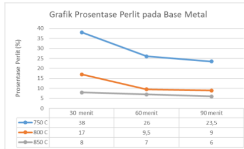
Gambar 5. 9 Perbandingan prosentase perlit pada base metal
