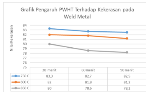
Gambar 5. 12 Grafik uji rockwell daerah weld metal
