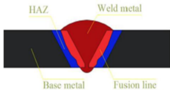
Gambar 2. 4 Penamaan zona dan batas pengaruh panas
