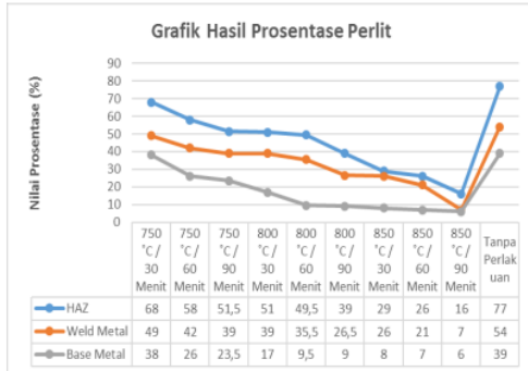
Gambar 5. 14 Grafik prosentase perlit pada struktur mikro
