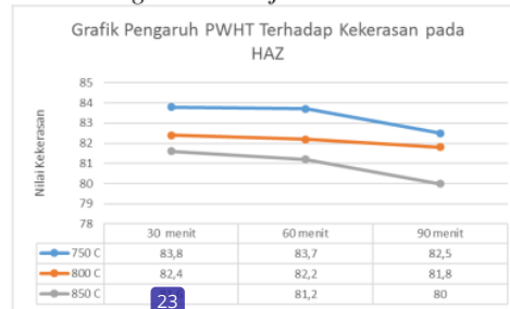
Gambar 5. 11 Grafik uji rockwell daerah HAZ
