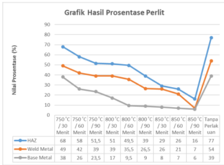
Gambar 5. 6 Grafik prosentase perlit
