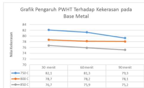
Gambar 5. 13 Grafik uji rockwell daerah base metal
