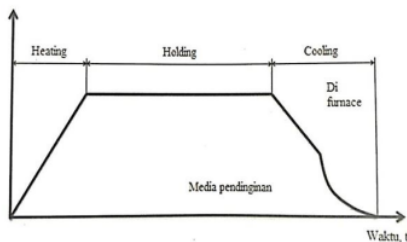
Gambar 2. 5 Siklus Termal PWHT
