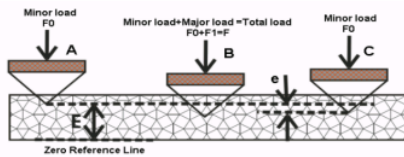
Gambar 2. 8 Penetrasi rockwell
