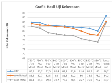
Gambar 5. 10 Grafik uji Kekerasan Rockwell
