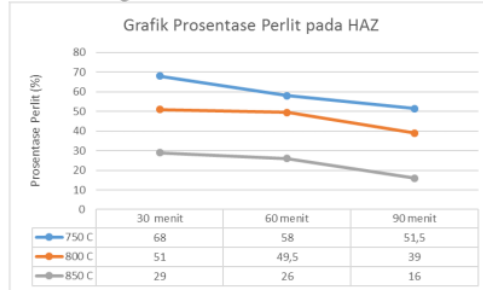
Gambar 5. 7 Perbandingan prosentase perlit pada HAZ
