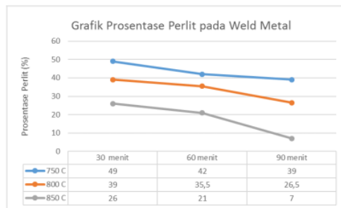
Gambar 5. 8 Perbandingan prosentase perlit pada weld metal
