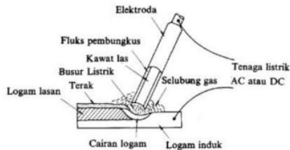
Gambar 2.1 Las busur dengan elektroda terbungkus
