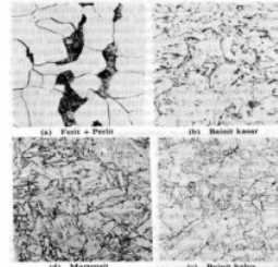
Gambar 2. 3 Mikrostruktur
