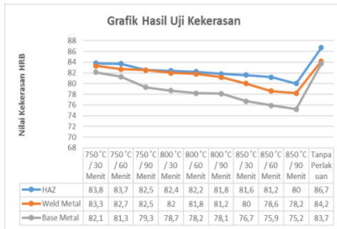
Gambar 5. 15 Grafik kekerasan pada uji kekerasan rockwell
