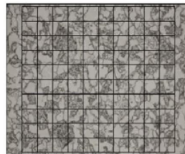
Gambar 2. 10 Perhitungan titik pada prosentase fasa
