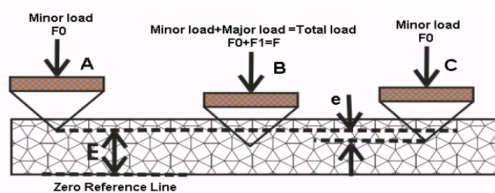
Gambar 2. 8 Penetrasi rockwell
