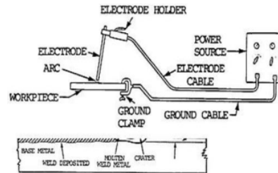
Gambar 2.1 Proses Las SMAW (Sumber : Harsono Wiryosumarto 2008)
