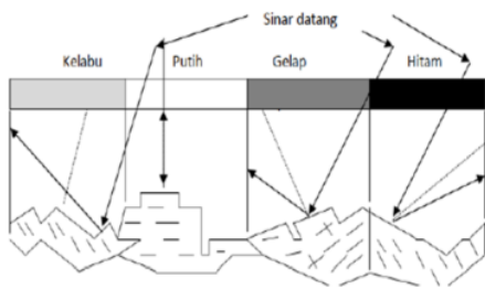
Gambar 2.6 Pantulan Sinar Uji Metalografi ( Sumber : Callister, 2004 )
