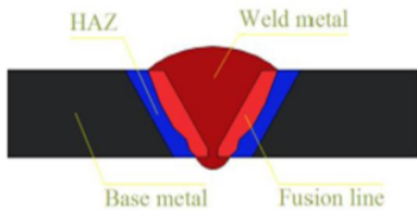
Gambar 2.3 Daerah Lasan
