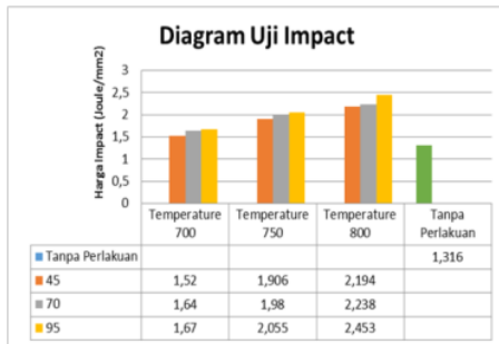
Gambar 4.9 Hasil Uji Impact
