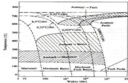
Gambar 2.2 Grafik CCT (Sumber : ASTM 43430)
