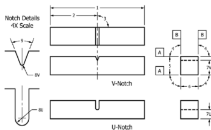
Gambar 3.6 Dimensi spesimen uji impact
