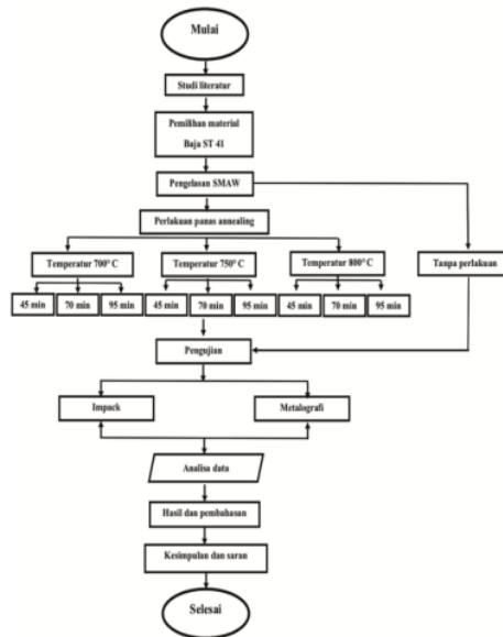
Gambar 3.1 Diagram Alir
