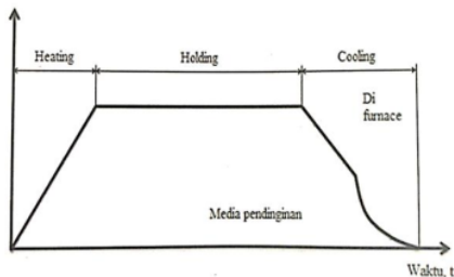
Gambar 2.4 Siklus Thermal PWHT
