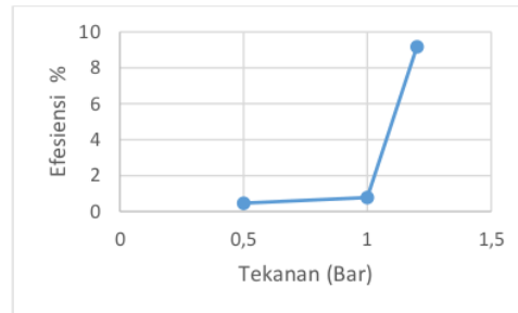
Grafik Tekanan Terhadap Efisiensi:
