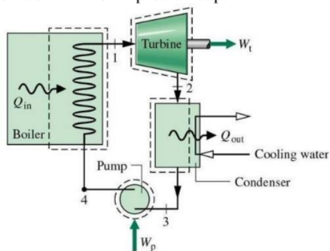
Gambar 1 Siklus Rankine
