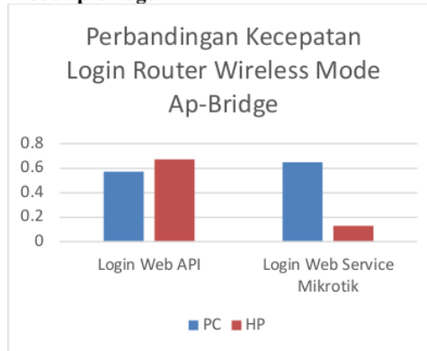
Gambar 3. 11 Kecepatan Login Router Mode ap-bridge
