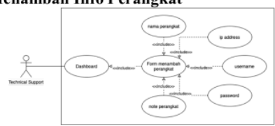
Gambar 2. 2 Use Case Tambah Perangkat
