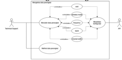
Gambar 2. 4 Use Case Rubah Konfigurasi
