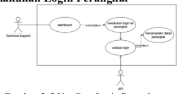
Gambar 2. 3 Use Case Login Perangkat
