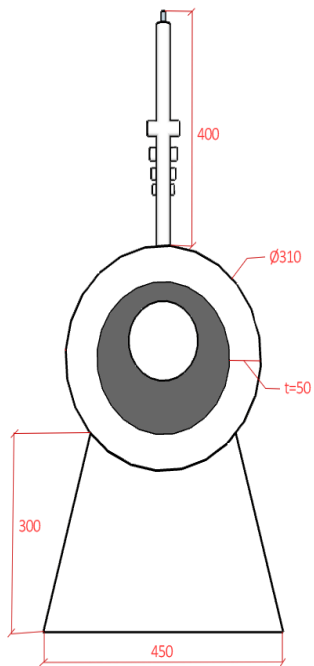
Tampak Depan
