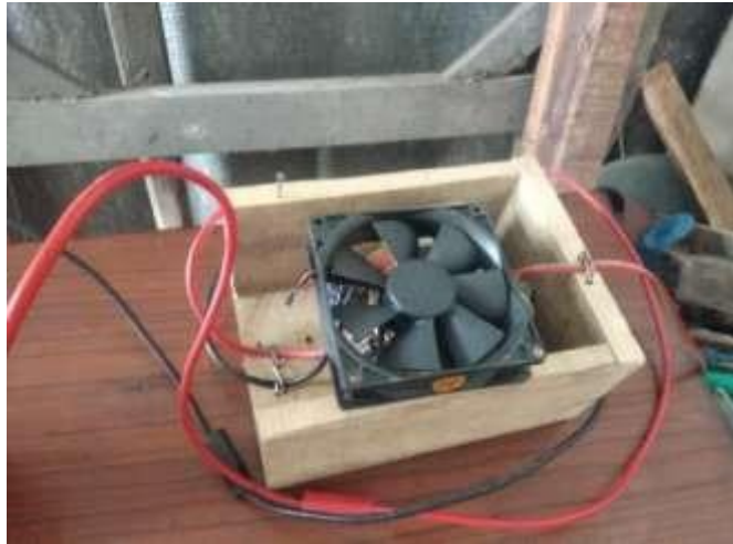
Gambar.Rangkaian Kipas pendingin dan travo multi arus
