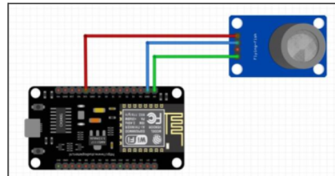
Gambar 20. Pengkabelan Gas Sensor
