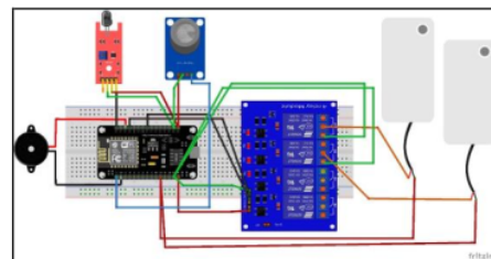
Gambar 21. Diagram Skematik Alat
