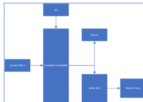
Gambar 1. Diagram Blok Alat
