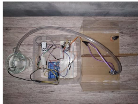
Gambar 33. Perakitan alat 1
