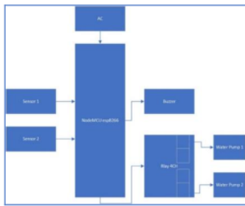
Gambar 18. Blok Diagram Alat
