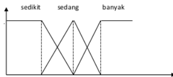
Gambar 11. Fungsi Keanggotaan MQ-2
