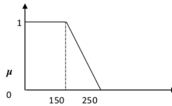
Gambar 12. Fungsi keanggotaan MQ-2 sedikit
