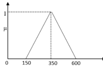
Gambar 17. Fungsi Keanggotaan Pompa on
