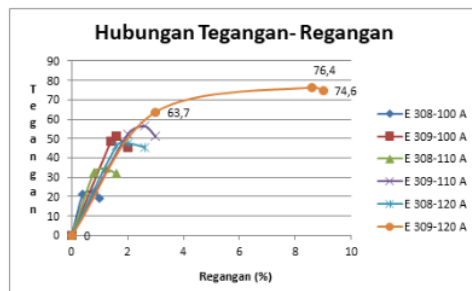
Gambar 13, Kurva hubungan Tegangan-Regangan
