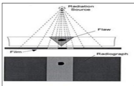
Gambar 5, Cara Kerja Radiografi
