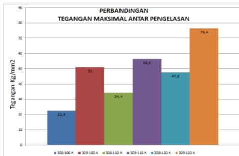
Gambar 14, Grafik Batang Tegangan Maksimal
