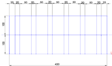
Gambar 2, Pembagian Ukuran Plat
