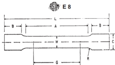
Gambar 6, Standar ASTM E8
