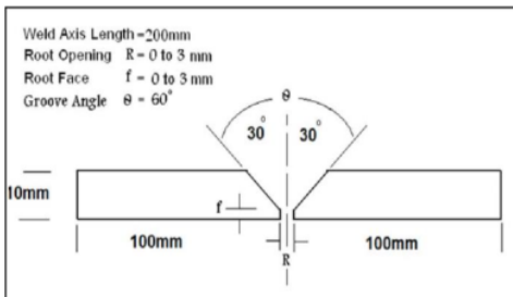
Gambar 3, V-Groove Yang digunakan
