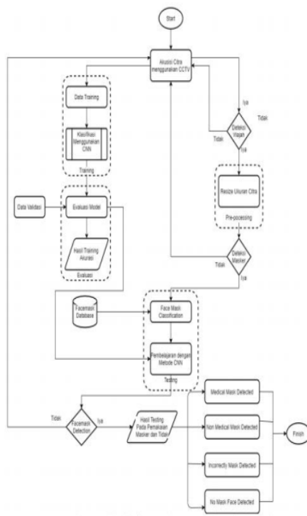
Gambar 1. Alur kerja sistem deteksi masker
