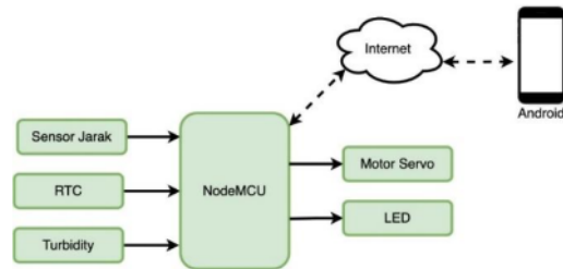
Gambar 2 Blok Diagram Alat Pakan Ikan
