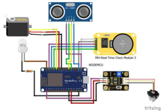
Gambar 3 Desain Rancang Alat
