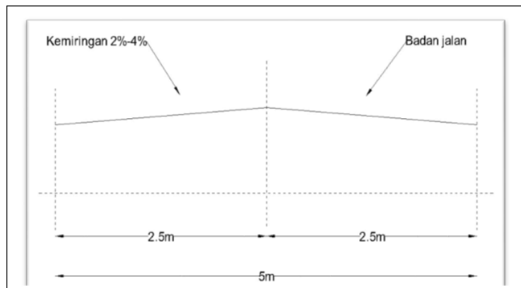
Gambar 4.1 Penampang Melintang Jalan
