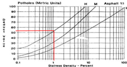
Gambar 4.2 Grafik Potholes
