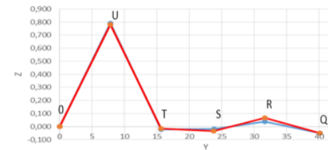
Gambar 6. Kedudukan titik-titik tampak samping kiri sebelum dan setelah T6 spesimen temperatur 400 0 dengan reduksi 5%
