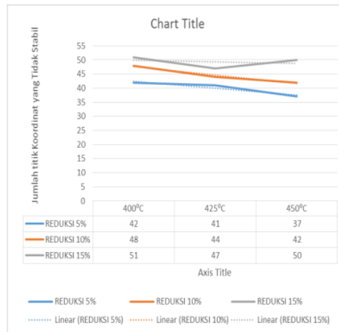
Gambar 8. Grafik pengaruh temperatur terhadap kestabilan titik-titik setiap spesimen
