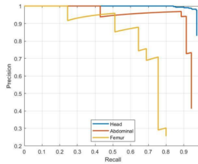
Gambar 6. Grafik precision/recall
