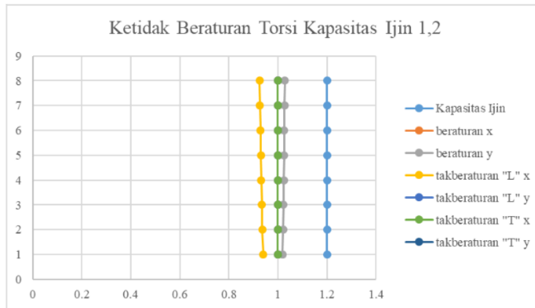
Gambar 3. 5 Grafik perbandingan Torsi dengan kapasitas ijin 1,2
