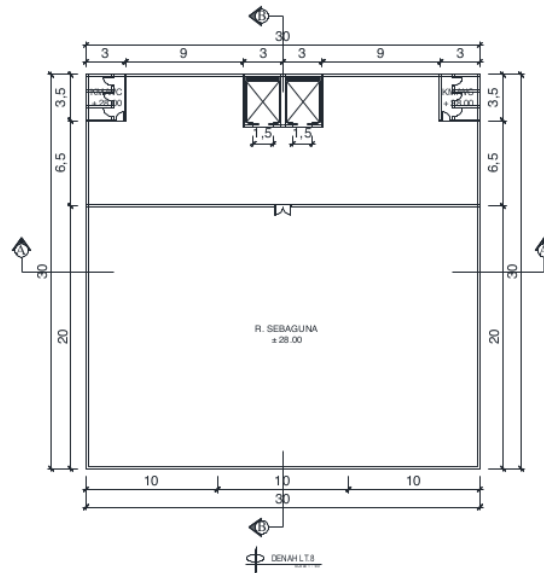
Gambar 2. 2 Denah bangunan beraturan
