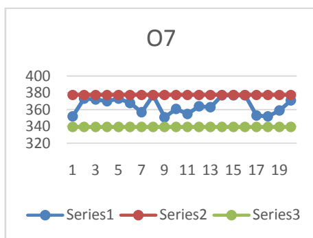
Peta Kontrol Keseragaman Data O7 Pemarut Kelapa
