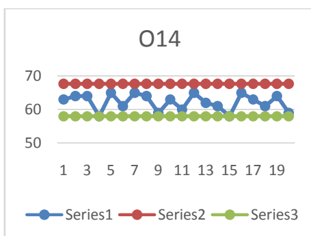
Peta Kontrol Keseragaman Data O14 Pemarut Kelapa
