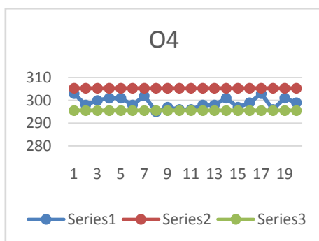
Peta Kontrol Keseragaman Data 04 Pencabut Bulu Ayam
