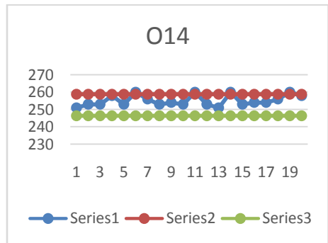
Peta Kontrol Keseragaman Data O14 Pencabut Bulu Ayam
