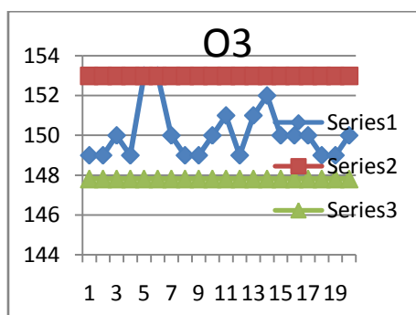
Peta Kontrol Keseragaman Data O3 Pemipil jagung
