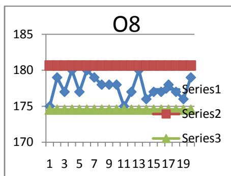
Peta Kontrol Keseragaman Data O8 Pemipil jagung
