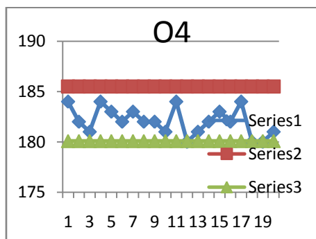
Peta Kontrol Keseragaman Data O4 Pemipil jagung
