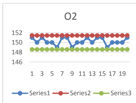
Peta Kontrol Keseragaman Data O2 Pencabut Bulu Ayam
