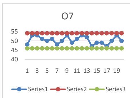
Peta Kontrol Keseragaman Data 07 Pencabut Bulu Ayam
