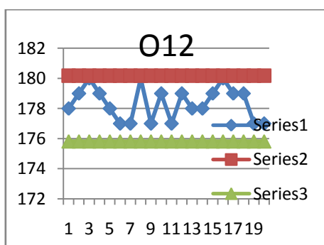
Peta Kontrol Keseragaman Data O12 Pemipil jagung
