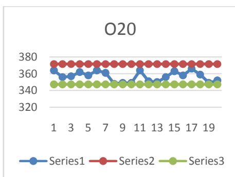
Peta Kontrol Keseragaman Data O20 Pemarut Kelapa
