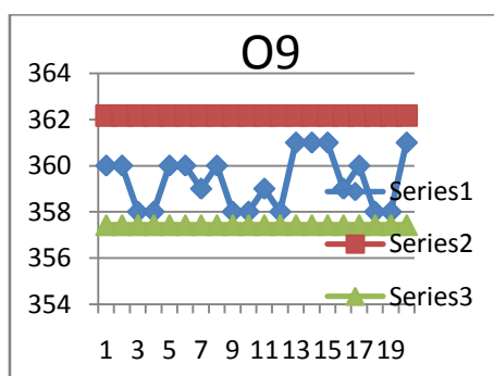
Peta Kontrol Keseragaman Data O9 Pemipil jagung
