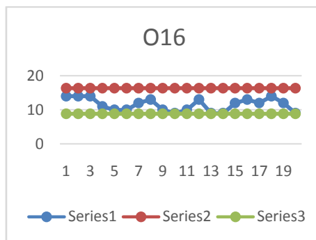
Peta Kontrol Keseragaman Data O16 Pemarut Kelapa
