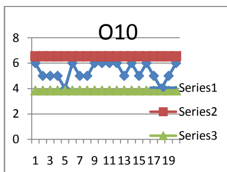
Peta Kontrol Keseragaman Data O10 Pemipil jagung
