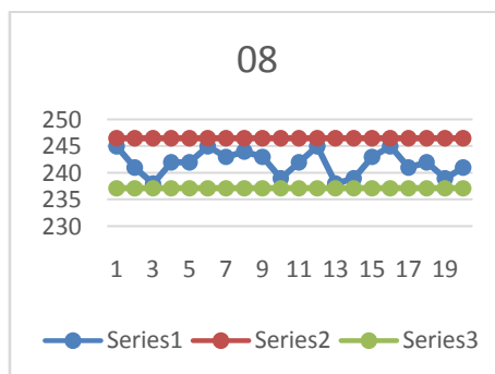
Peta Kontrol Keseragaman Data 08 Pencabut Bulu Ayam
