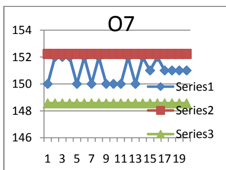
Peta Kontrol Keseragaman Data O7 Pemipil jagung
