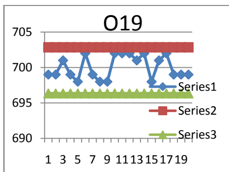
Peta Kontrol Keseragaman Data O19 Pemipil jagung
