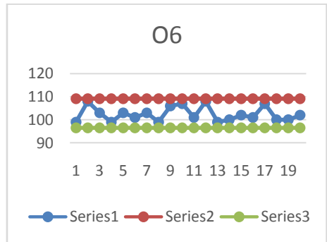
Peta Kontrol Keseragaman Data O6 Pemarut Kelapa
