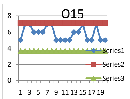
Peta Kontrol Keseragaman Data O15 Pemipil jagung
