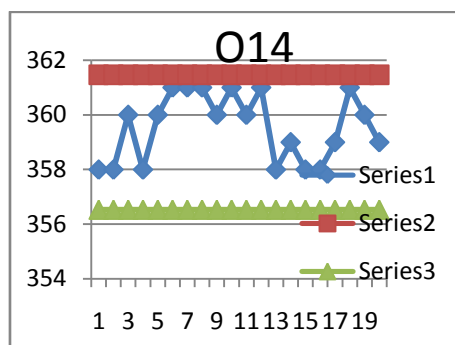
Peta Kontrol Keseragaman Data O14 Pemipil jagung
