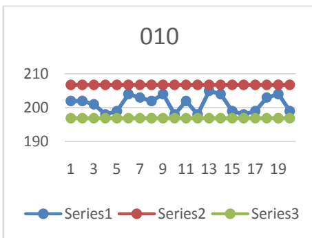
Peta Kontrol Keseragaman Data O10 Pencabut Bulu Ayam
