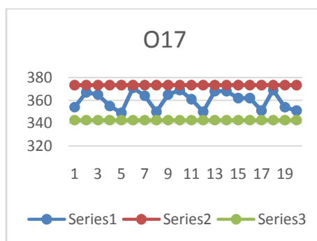
Peta Kontrol Keseragaman Data O17 Pemarut Kelapa
