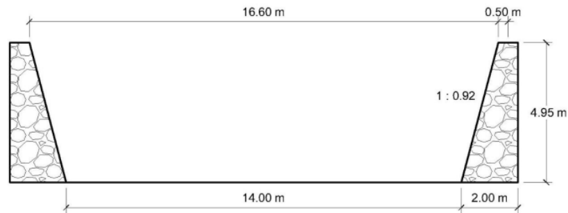
Gambar 3.3 Evaluasi Penampang Periode 10 tahun
