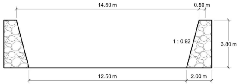
Gambar 3.1 Evaluasi Penampang Periode 2 tahun
