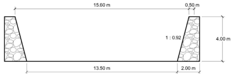
Gambar 3.2 Evaluasi Penampang Periode 5 tahun
