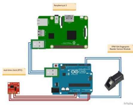
Gambar 2.3. Alur Komunikasi sistem
