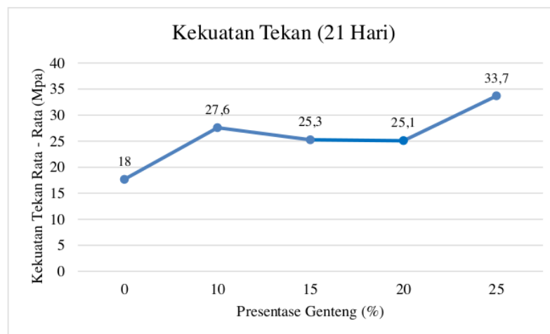
Gambar 4 Kekuatan Tekan Beton Alir Pada Umur 21 Hari
