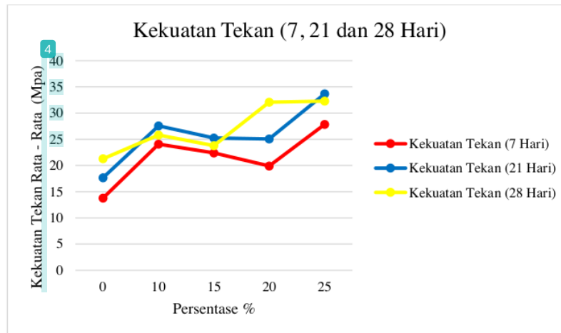
Gambar 6 Kekuatan Tekan Beton Alir Gabungan
