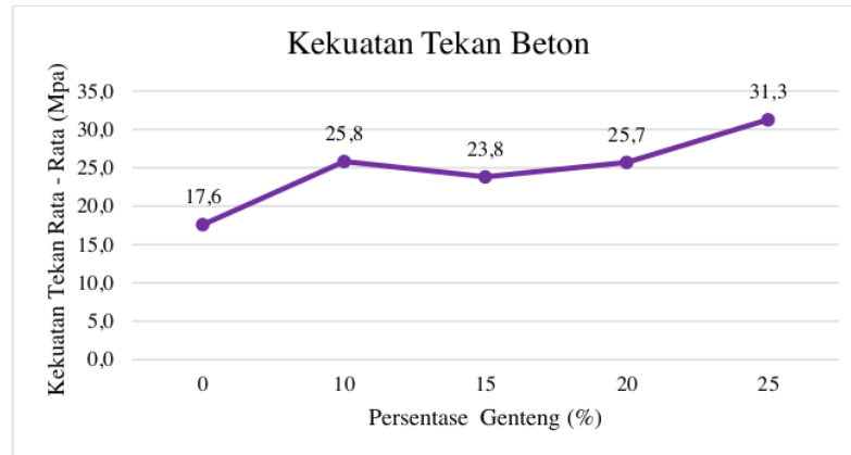
Gambar 8 Kekuatan Tekan Beton Alir Rata - Rata
