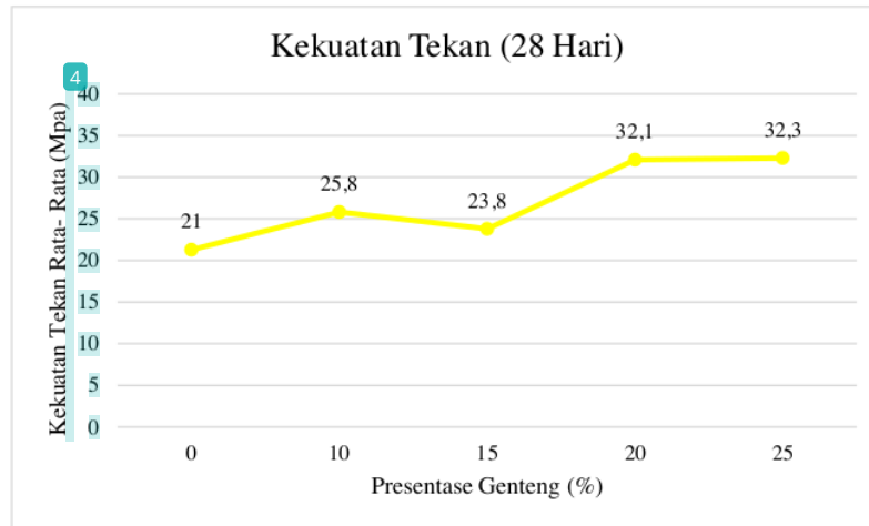
Gambar 5 Kekuatan Tekan Beton Alir Pada Umur 28 Hari
