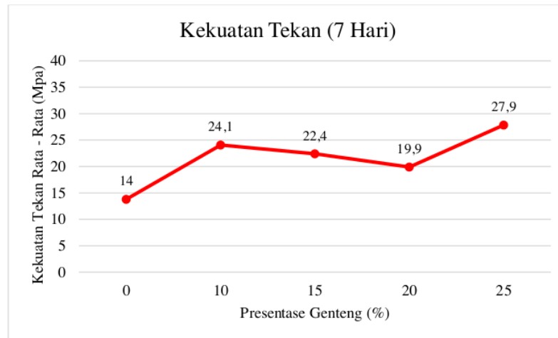
Gambar 3 Kekuatan Tekan Beton Alir Pada Umur 7 Hari
