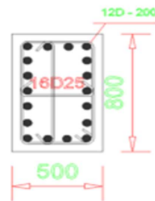
Gambar 4.5 Kolom
