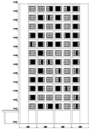
Gambar 4.1 Potongan A-A Apartemen
