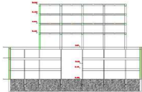
Gambar 4.8 Galian Tanah Metode Top-Down (Sumber : Kajewski 1994)
