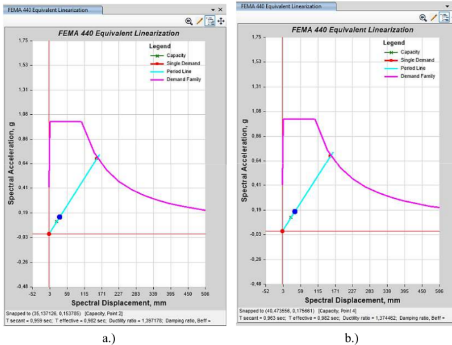
Gambar 5 a.) Hasil nilai kalkulasi grafik kurva kapasitas arah-X SRPMK, b.) Hasil nilai kalkulasi grafik kurva kapasitas arah-Y SRPMK.
