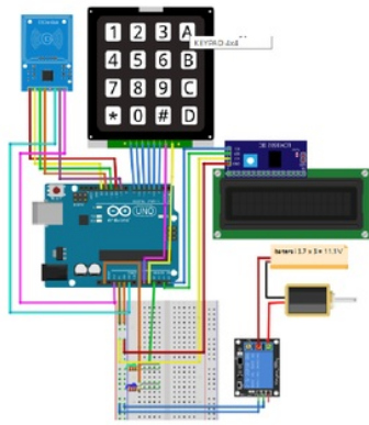
Gambar 9. Perancangan Rangkaian Alat
