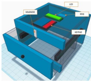
Gambar 8. Desain Alat
