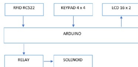
Gambar 6. Diagram Blok Sistem
