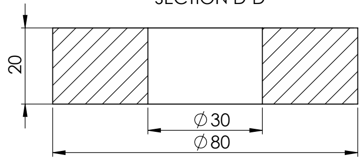
SECTION D-D
