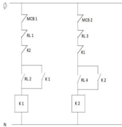
Gambar 6. Rangkaian Control
