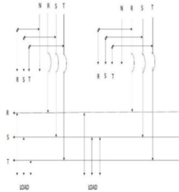
Gambar 7. Rangkaian Utama Gardu
