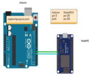
Gambar 2. Rangkaian Arduino ke NodeMCU
