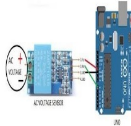
Gambar 4. Rangkaian Arduino ke Sensor ZMPT101B
