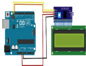
Gambar 3. Rangkaian Arduino ke LCD
