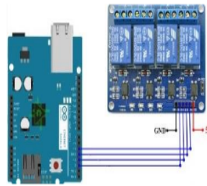
Gambar 1. Rangkaian Arduino ke relay
