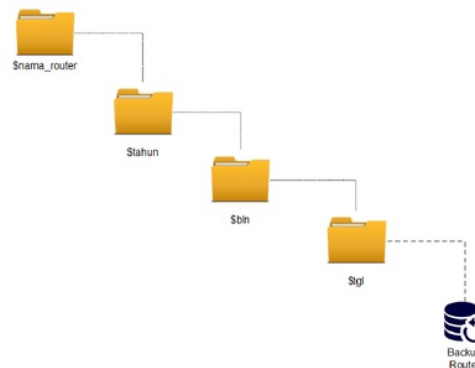
Gambar 13. Struktur folder Direktori Penyimpanan
