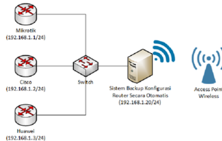
Gambar 17. Skenario Pengujian Sistem
