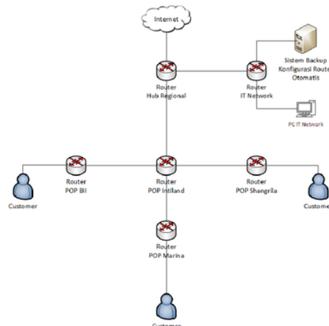
Gambar 5. Perancangan Arsitektur Jaringan
