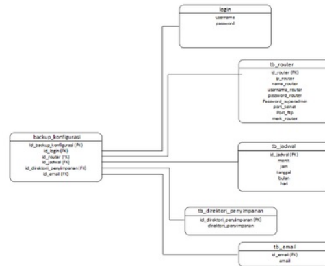
Gambar 12. ERD Backup Konfigurasi Router
