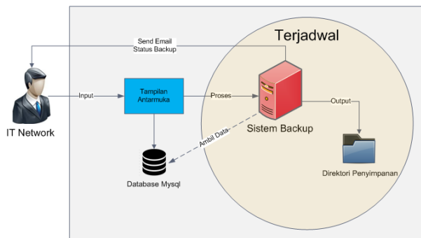
Gambar 6. Alur kerja Sistem
