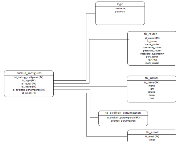
Gambar 12. ERD Backup Konfigurasi Router
