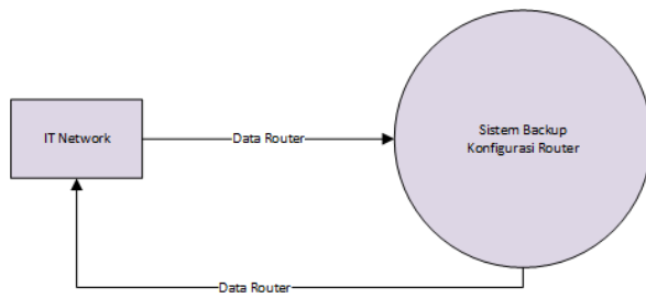
Gambar 10. Diagram Konteks Sistem Backup Konfigurasi Router
