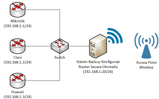
Gambar 17. Skenario Pengujian Sistem
