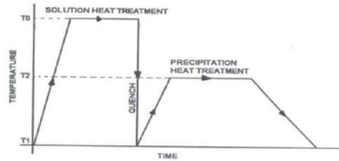
Gambar 2. Siklus Perlakuan Panas T6.
