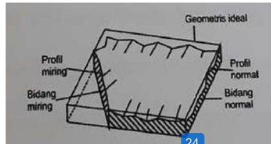
Gambar 3. Bidang dan profil permukaan.
