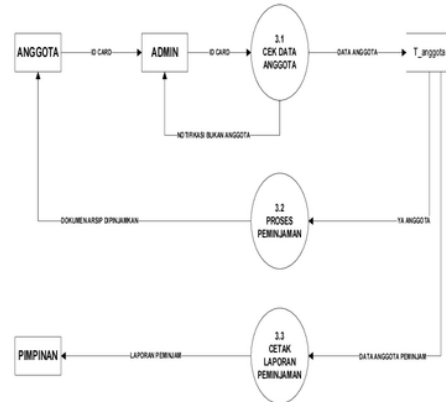
Gambar 11. DFD Level 2 Proses Peminjaman Arsip
