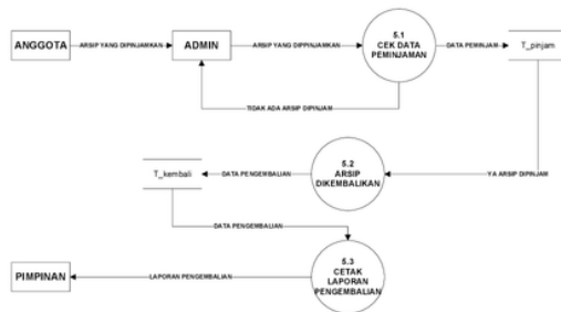
Gambar 13. DFD Level 2 Proses Pengembalian Arsip
