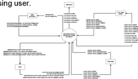
Gambar 7. Diagram Konteks / DFD Level 0 Sistem Aplikasi Arsip
