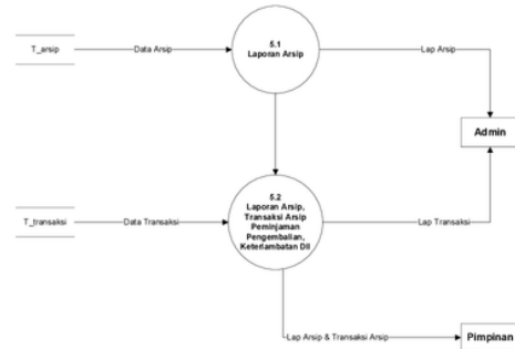
Gambar 14. DFD Level 2 Proses Laporan Arsip & Transaksi Arsip
