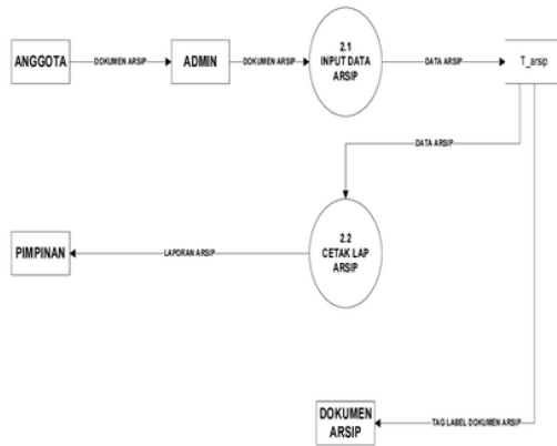
Gambar 10. DFD Level 2 Proses Pengarsipan
