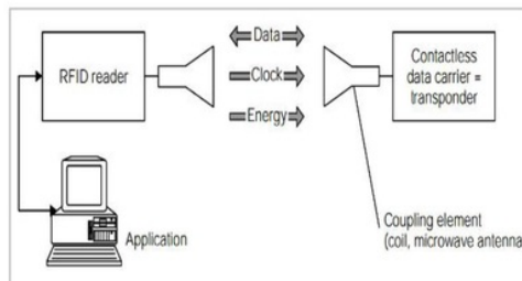
Gambar 1. Komponen sistem RFID (Finkenzeller 2003)
