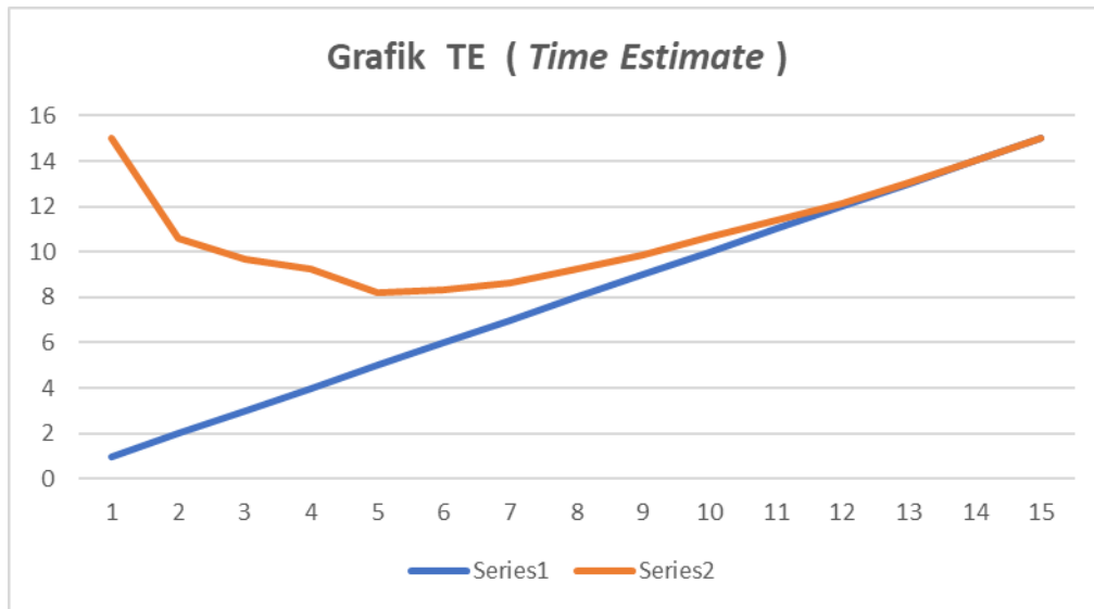
Gambar4.6Grafik TE
