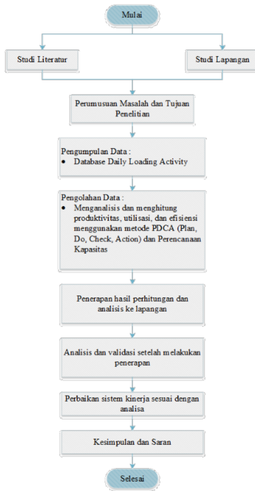
Gambar 3 Metodologi Penelitian
