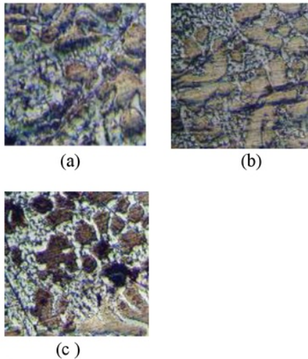
Gambar 5. (a). Temperatur penguangan 600°C kodefikasi A' temperatur cetakan suhu kamar. (b). Temperatur penguangan 650°C kodefikasi A' temperatur cetakan suhu kamar. (c). Temperatur penguangan 700°C kodefikasi A' temperatur cetakan suhu kamar.
