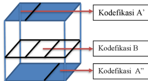
Gambar 1. Kodefikasi spesimen
