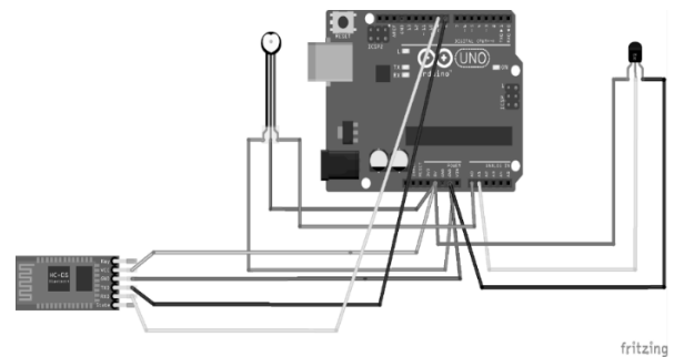
Gambar 3 Rangkaian Keseluruhan
