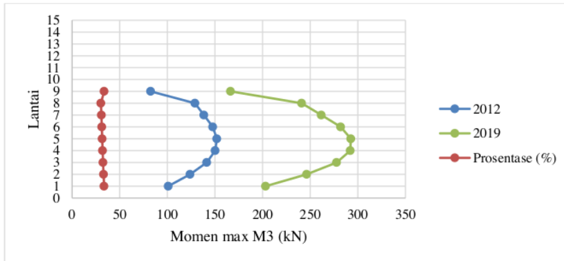
Gambar 14 Grafik perbandingan momen pada balok B61 SNI:2019 dan SNI:2012
