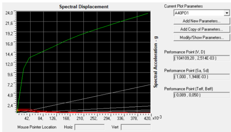
Gambar 12 Base Shear dan Displacement arah x-x
