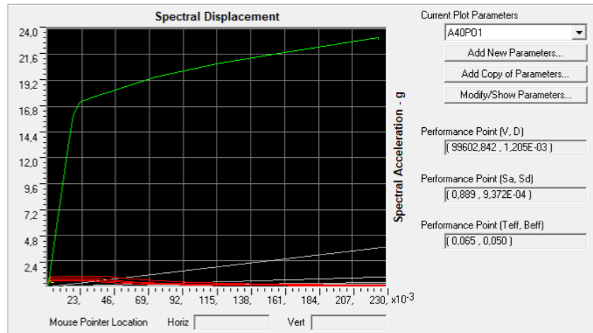
Gambar 11 Base Shear dan Displacement arah y-y
