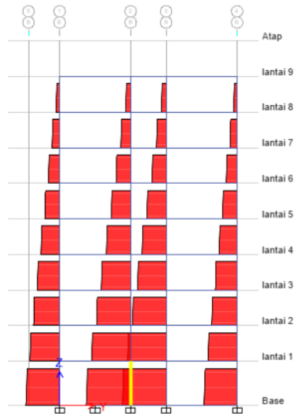
Gambar 8 Momen balok B61
