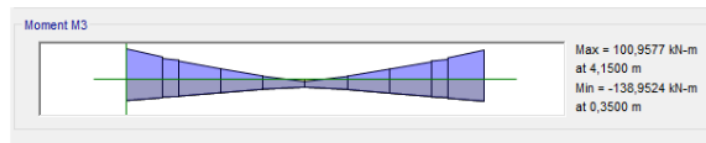
Gambar 7 Momen balok B61
