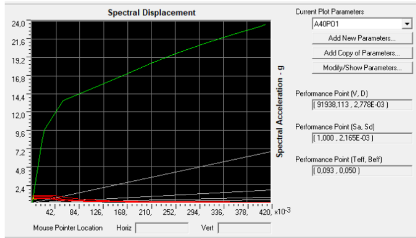
Gambar 13 Base Shear dan Displacement arah y-y
