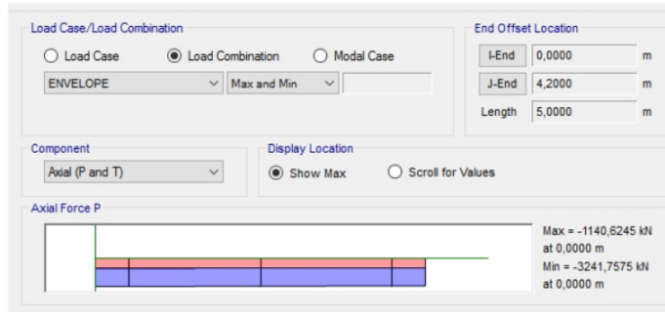
Gambar 9 Aksial Momen Momen kolom c10
