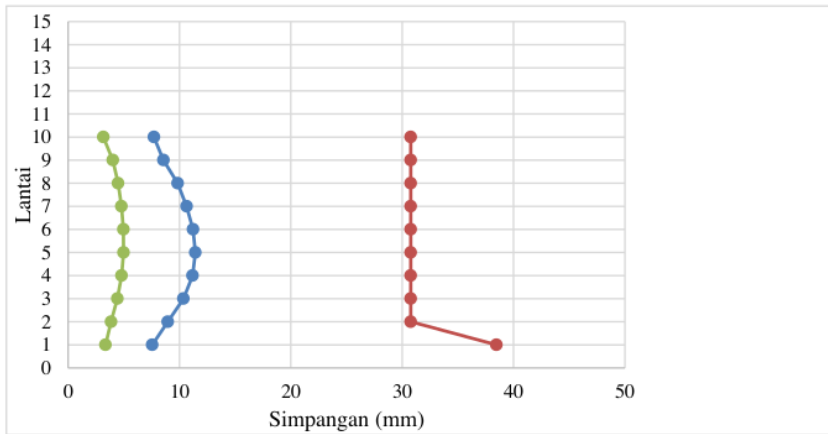
Gambar 10 Grafik simpangan x dan y
