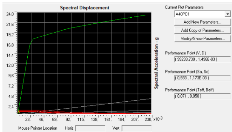
Gambar 11 Base Shear dan Displacement arah x-x
