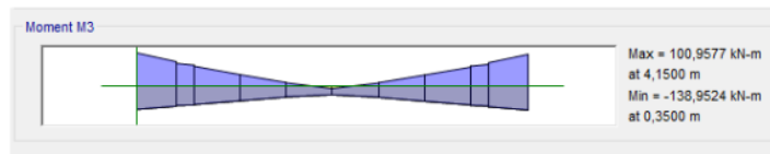
Gambar 4 Momen balok B61
