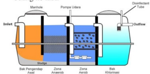
Gambar: Penerapan Utilitas Air Kotor
