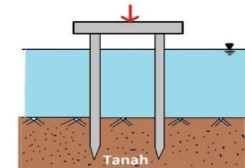
Gambar: Penerapan Tiang Pancang Beton
