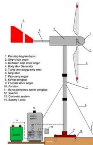
Gambar: Penerapan Instalasi Listrik
