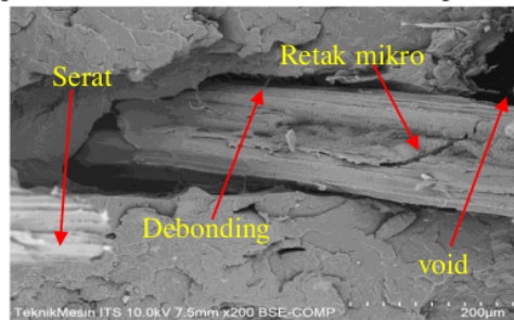
Gambar 4.8. Hasil pengujian SEM Spesimen dengan ukuran mesh 250-300 variasi serat
