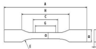
Gambar. 5 Spesifikasi spesimen ASTM D 638-01
