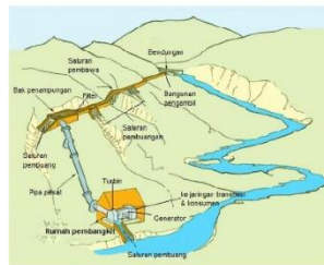
Gambar 2. Skema PLTMH
