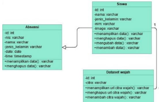
Gambar 10. Class Diagram Sistem Absensi Pengenalan Wajah
