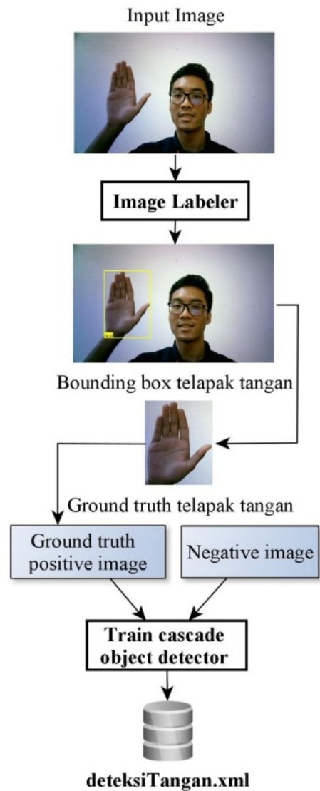
Gambar.2 Proses Pembelajaran Deteksi Telapak Tangan
