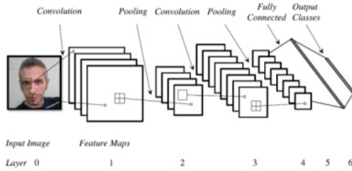
Gambar 6. Arsitektur CNN [13]
