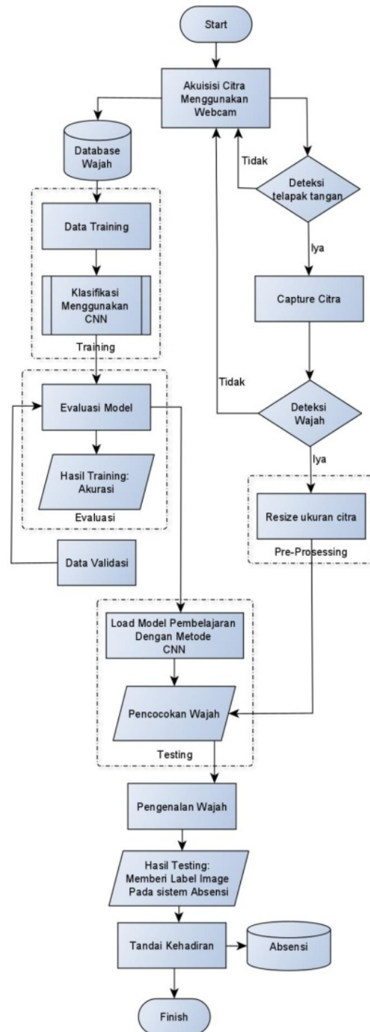
Gambar.1 Alur kerja sistem absensi cerdas
