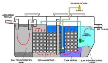
Gambar 6. Sistem IPAL
