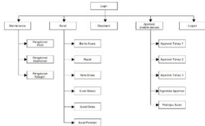
Gambar 6 Struktur Menu
