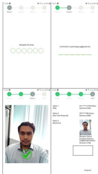
Gambar 17 Implementasi MFA
