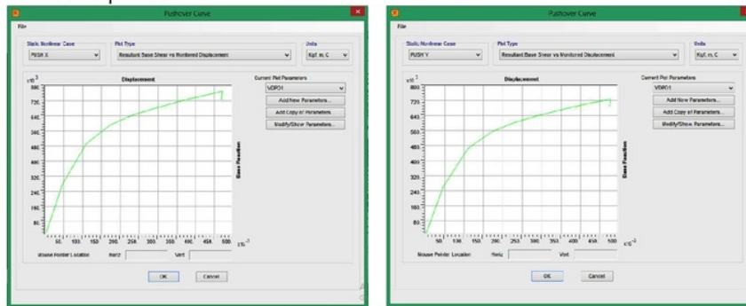
Gambar 4. 2 kurva kapasitas x dan y (Sumber: Hasil SAP2000)
