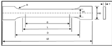
Gambar. 3. Spesifikasi cetakan ASTM D 638 -02
