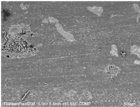
Gambar 10. SEM Komposit Polypropylane dengan penguat abu dasar ukuran 100-150 mesh dan serat dengan panjang 3 mm, putaran 750 Rpm dengan waktu pengadukan 60 menit.
