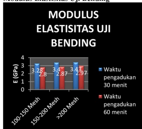
Gambar 8. Grafik modulus elastisitas
