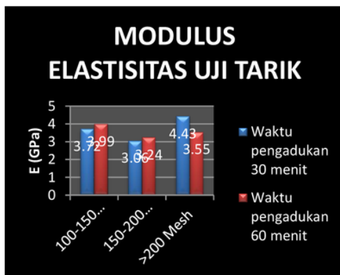
Gambar 6. Grafik modulus elastisitas uji tarik.
