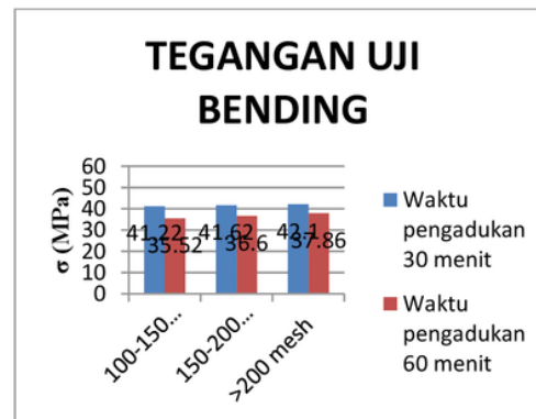
Gambar 7. Grafik tegangan uji bending
