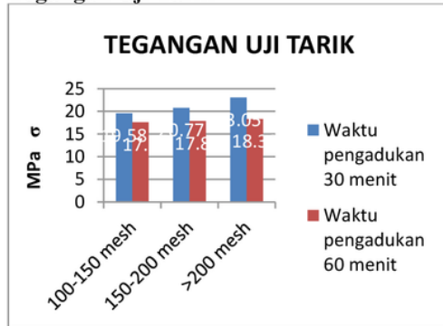
Gambar 4. grafik tegangan uji tarik
