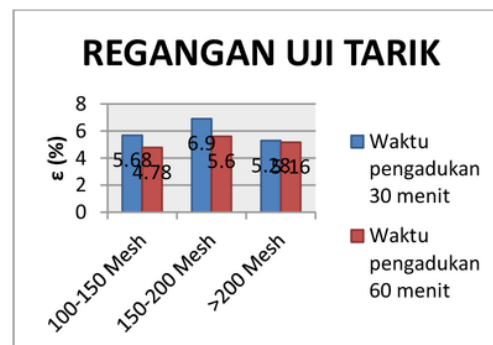
Gambar 5. Grafik regangan uji tarik
