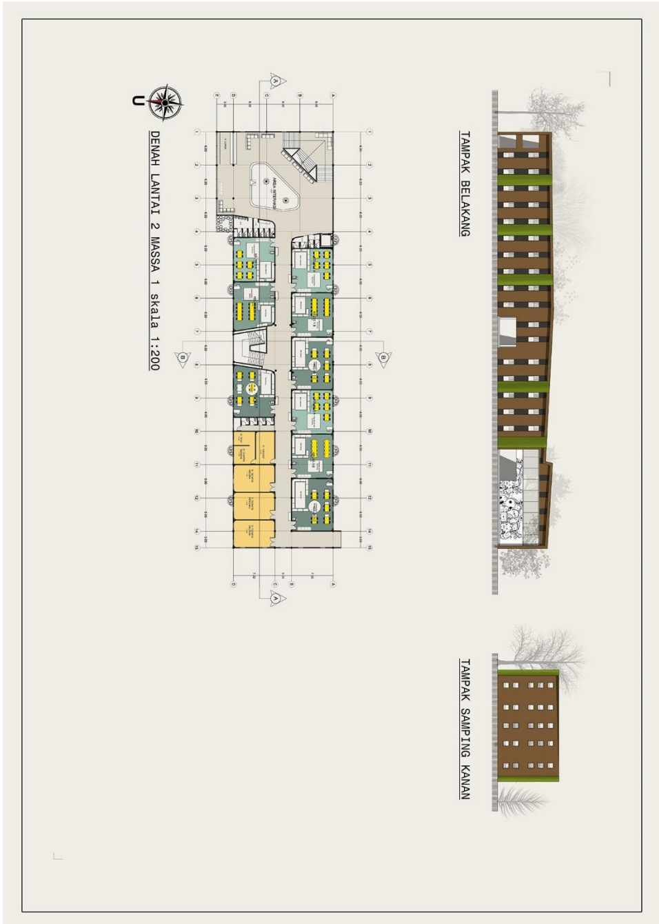
Gambar 1.28 Denah Lt.2 dan tampak potongan massa 1
