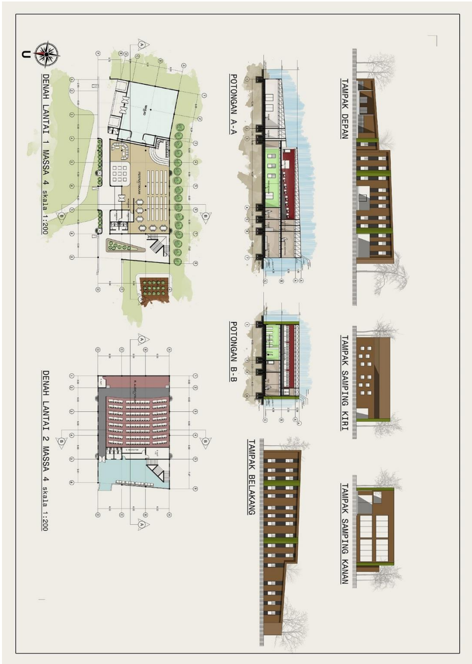
Gambar 1.32 Denah Lt 1 dan tampak potongan massa 4
