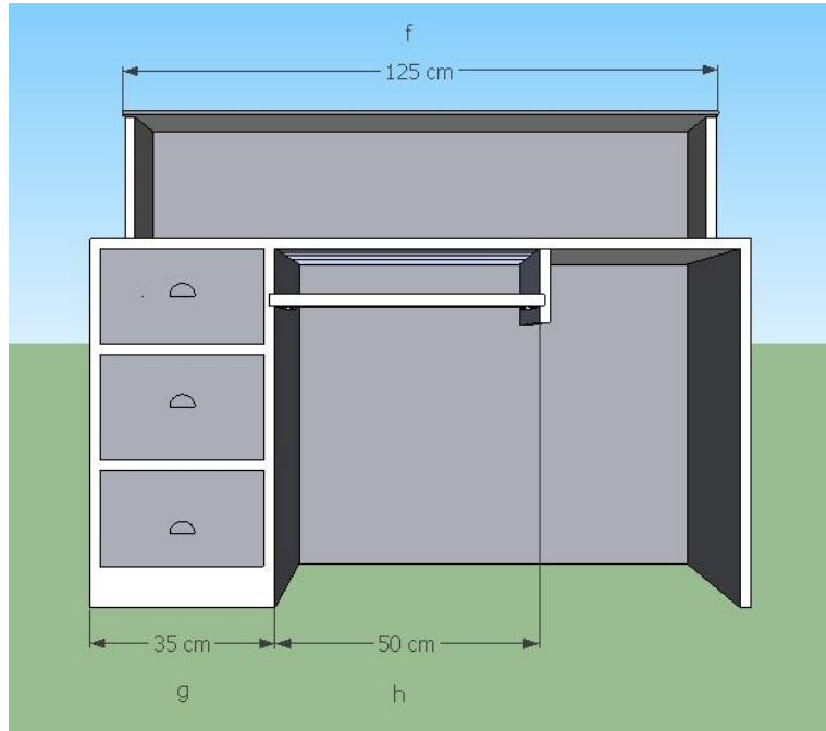
LAMPIRAN 2.1. Gambar 1 dimensi meja teller setelah perbaikan (tampak depan)
