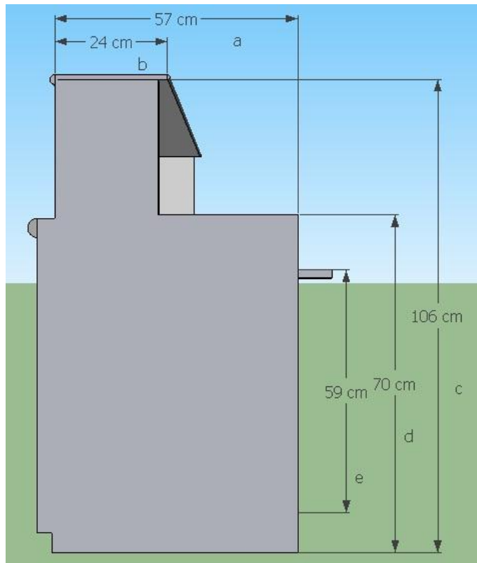
LAMPIRAN 2.2. Gambar 2 dimensi meja teller setelah perbaikan (tampak samping)
