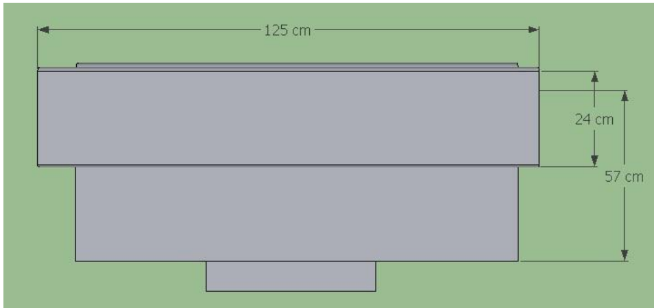
LAMPIRAN 2.4. Gambar 4 dimensi meja teller setelah perbaikan (tampak belakang)
