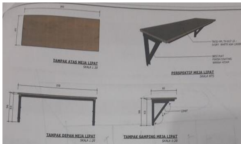
Gambar 6 Sketsa Produk Meja Lipat.
