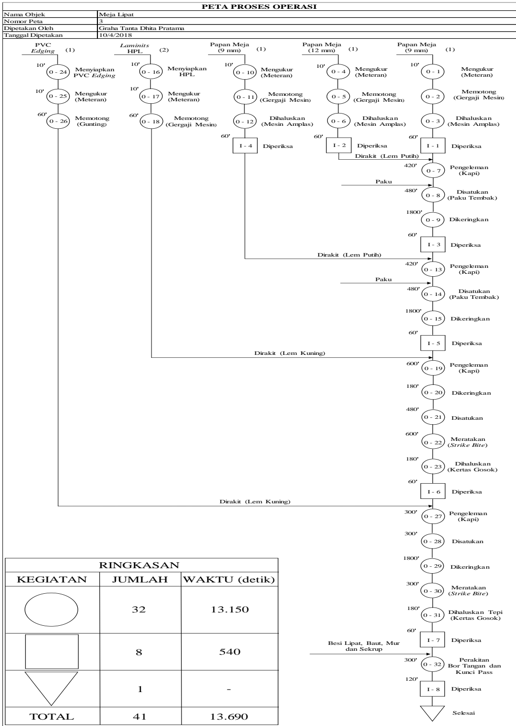
Gambar 14 Peta Proses Operasi Meja Lipat.
