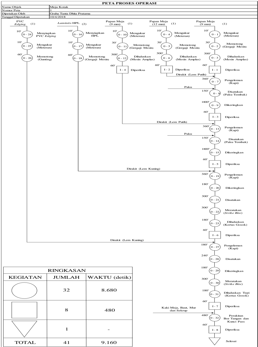
Gambar 12 Peta Proses Operasi Meja Kotak.
