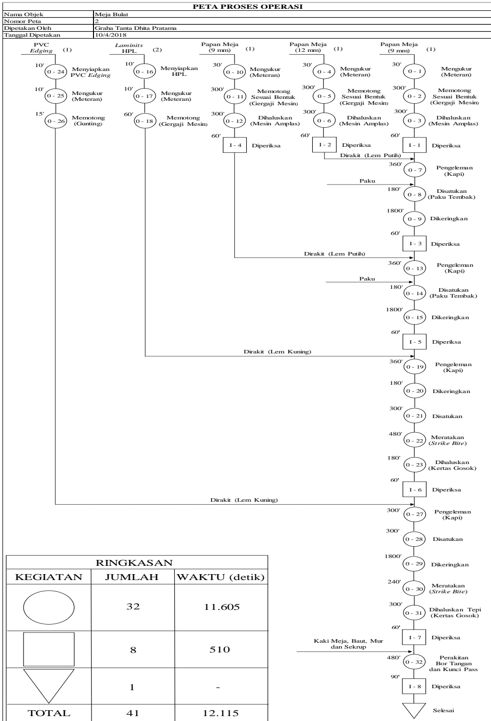
Gambar 13 Peta Proses Operasi Meja Bulat.
