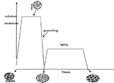
Gambar 2. Siklus Perlakuan Panas T6
