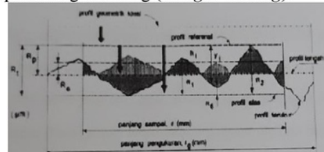
Gambar 6. Profil Kekasaran Permukaan
