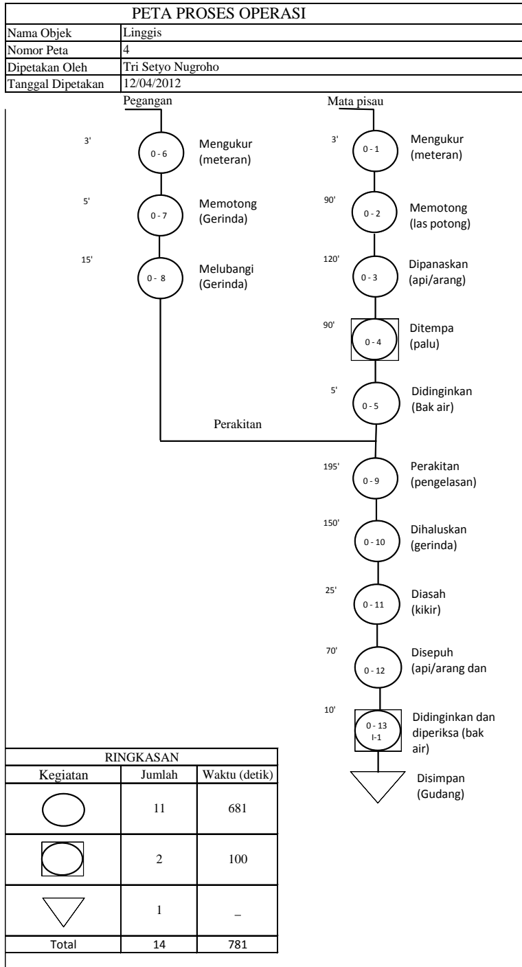
Gambar 10 peta proses operasi linggis
