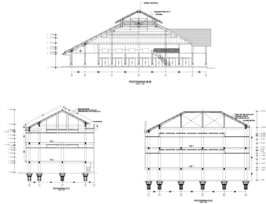
Gambar Potongan Gedung Serba Guna
